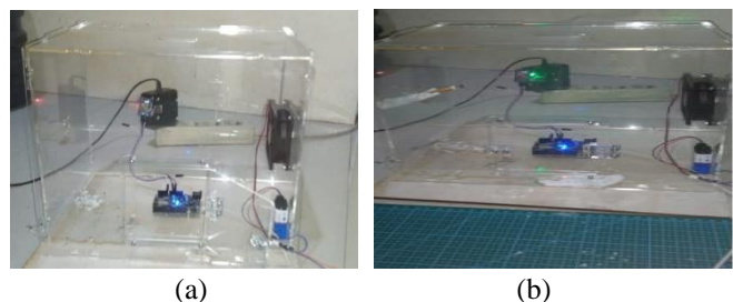
Gambar 16 (a) Pengujian Sensor MQ 135 tanpa asap, (b) Pengujian Sensor MQ 135 dengan asap rokok
