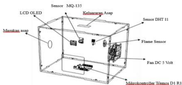
Gambar 8 Gambar Perancangan Prototype.
